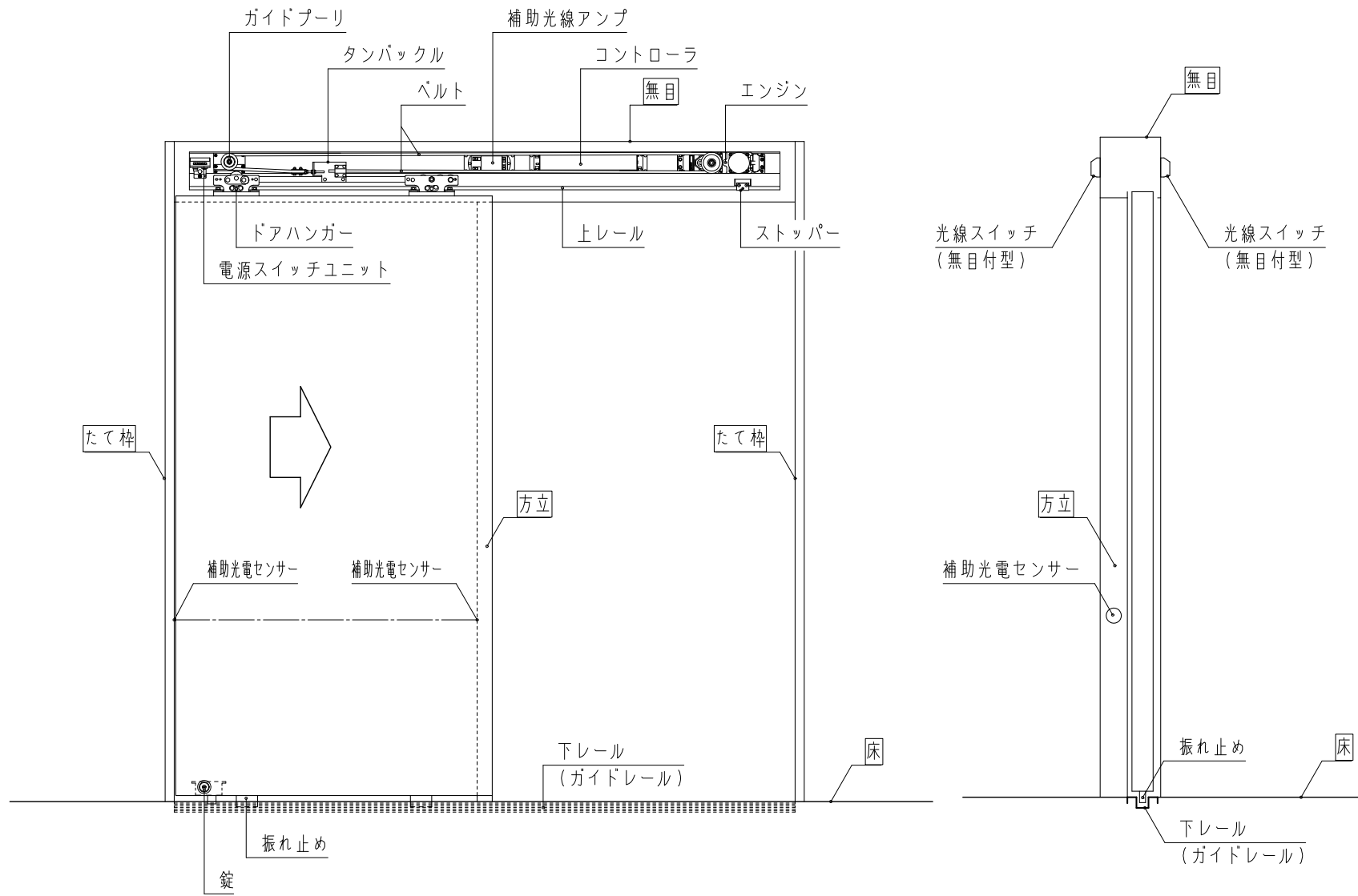
(片引き自動ドア各部の名称)
