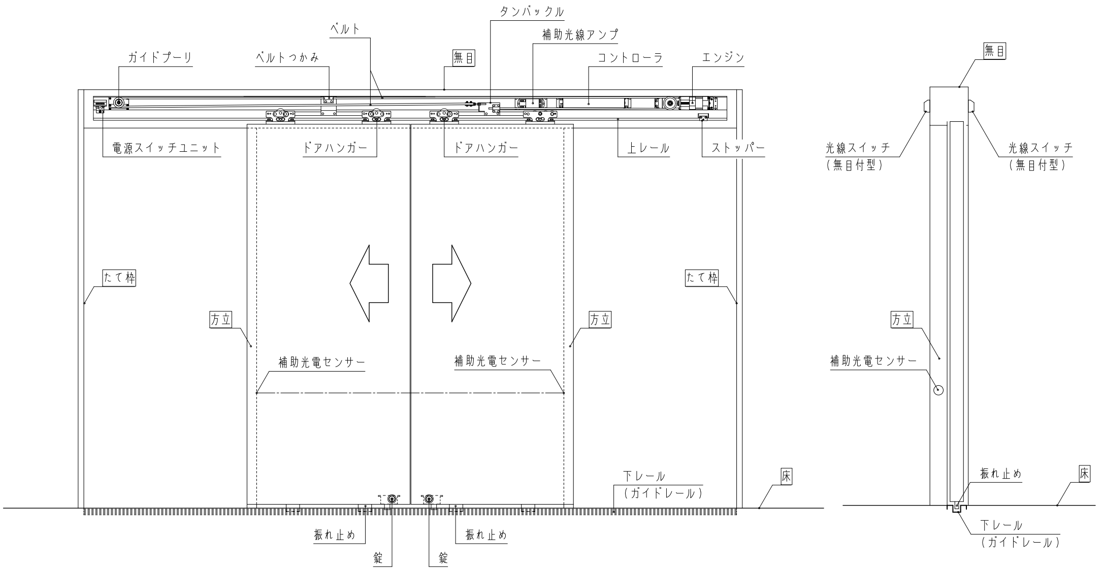
(引分け自動ドア各部の名称)
